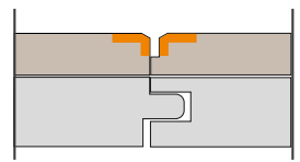
bisello e battente | bevel and groove
