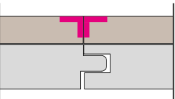
spigolo vivo | square edge
