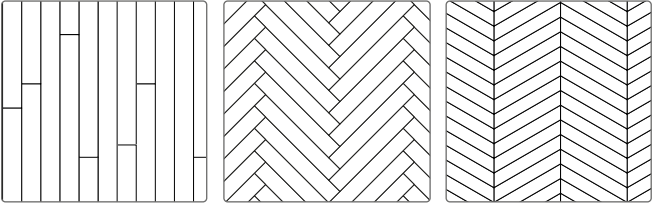
A CORRERE REGULAR INSTALLATION SPINA ITALIANA 90° HERRINGBONE 90° PUNTO D'UNGHERIA 60° CHEVRON 60°
