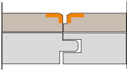
bisello e battente | bevel and groove
