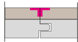
spigolo vivo | square edge
